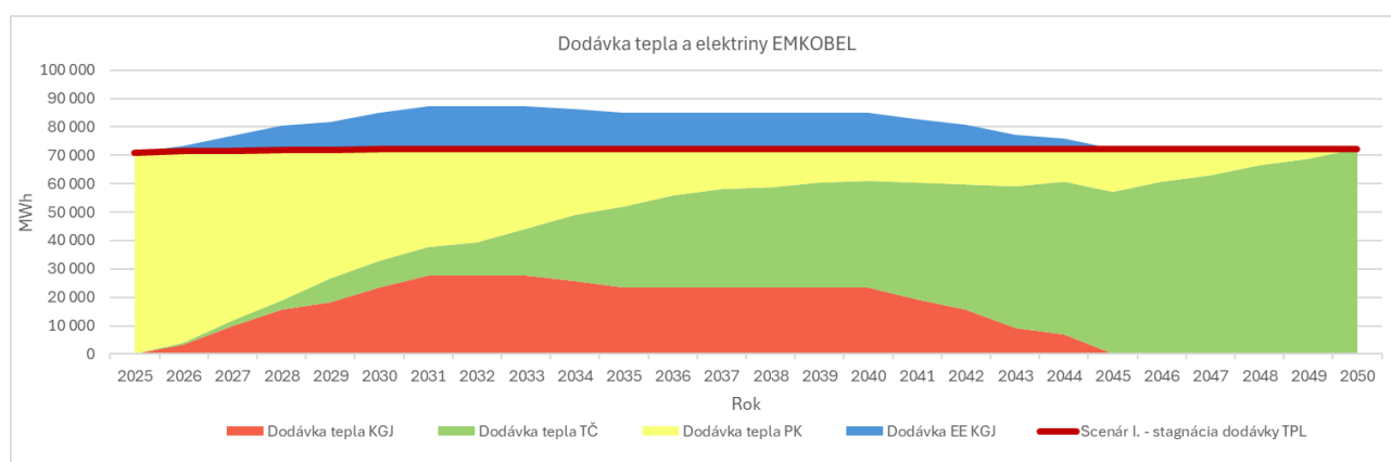
Obr. 48: Dodávka tepla a elektriny EMKOBEL – scenár 1 stagnačný
