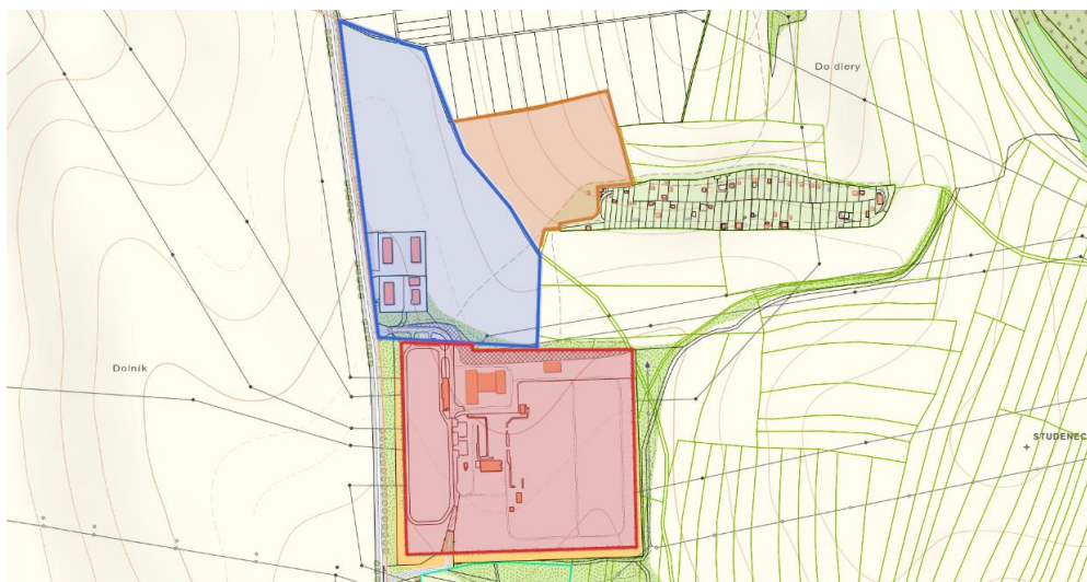
Obr. 40: Umiestnenie FVE
