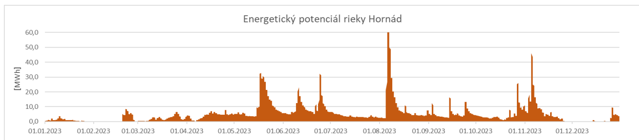
Obr. 43: Energetický potenciál rieky Hornád počas roka (MWh)
