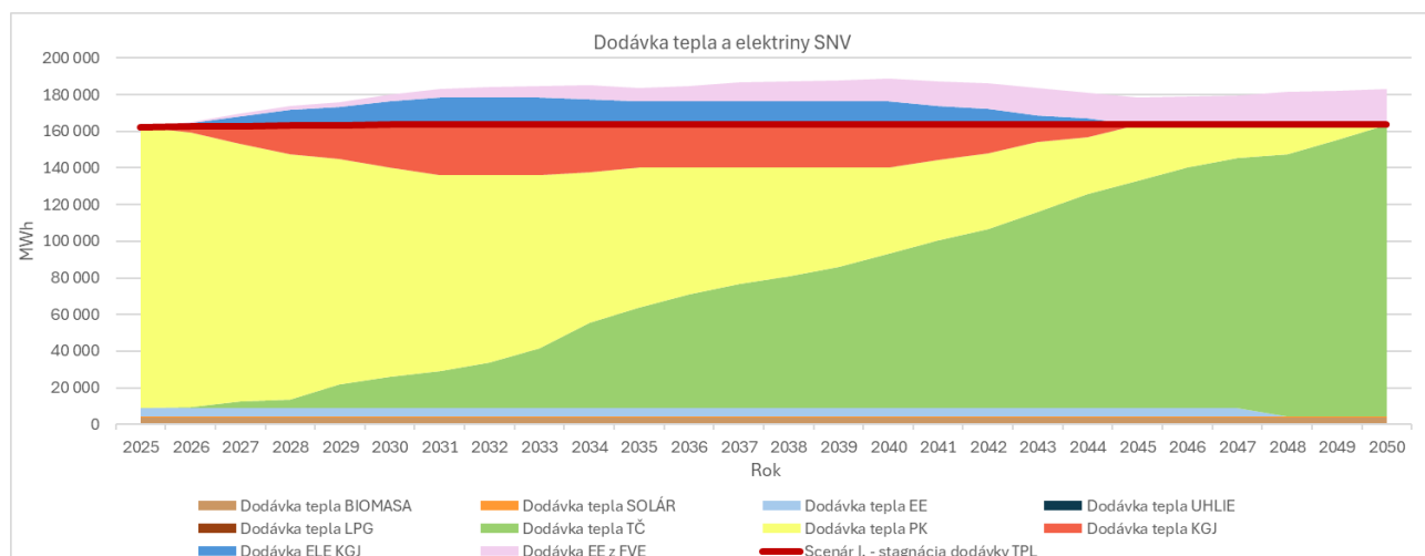
Obr. 55: Energetické vstupy - celá SNV - scenár 1 stagnačný
