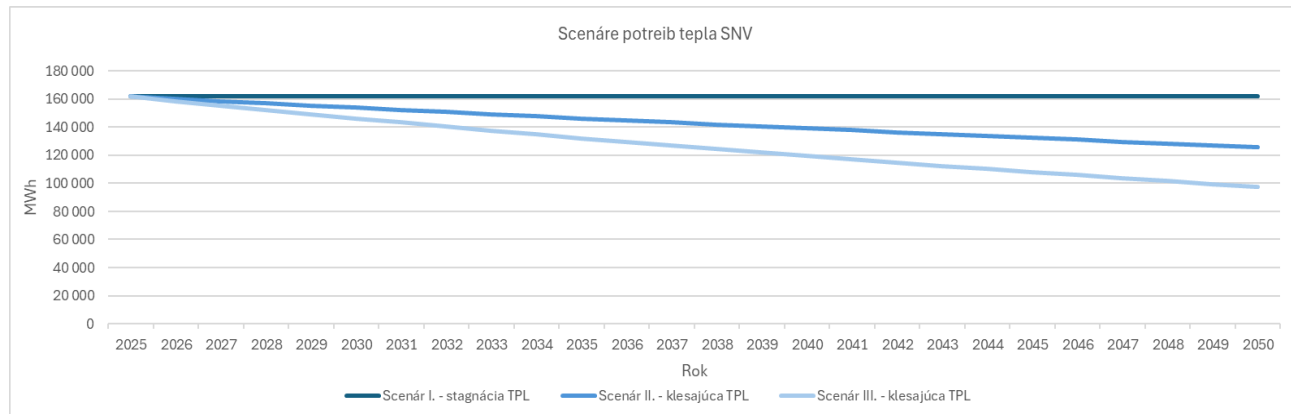
Obr. 46: Grafické znázornenie scenárov potrieb tepla
