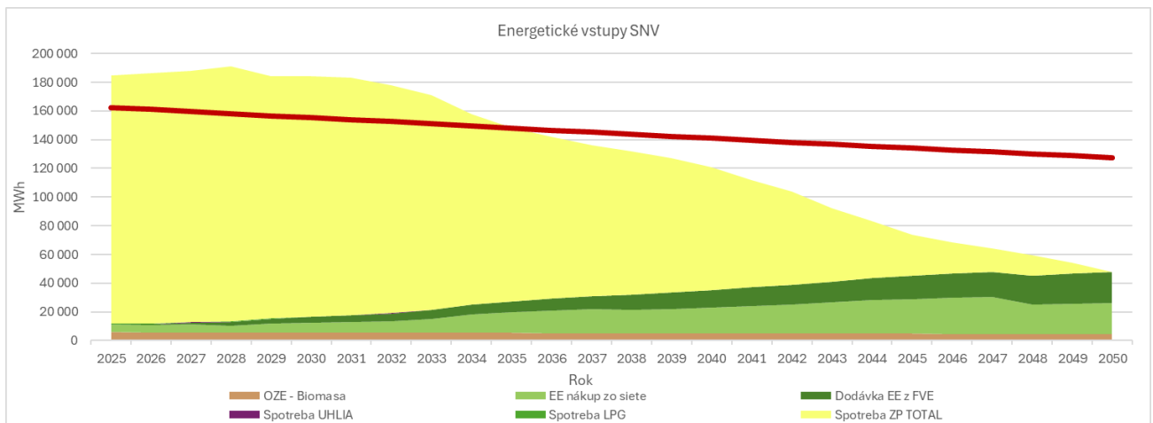
Obr. 67: Energetické vstupy - celá SNV - scenár 2 klesajúci o 1%
