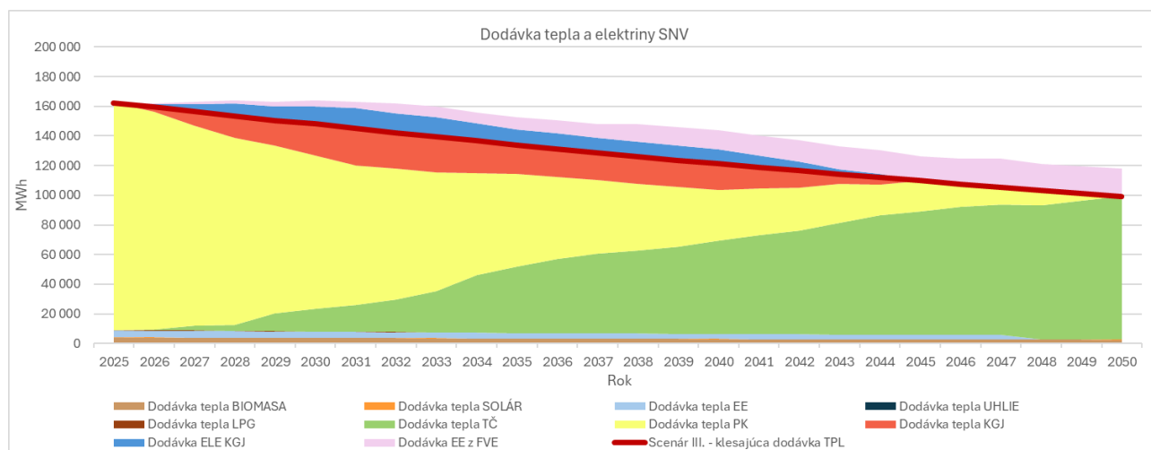
Obr. 79: Energetické vstupy - celá SNV - scenár 3 klesajúci o 2%
