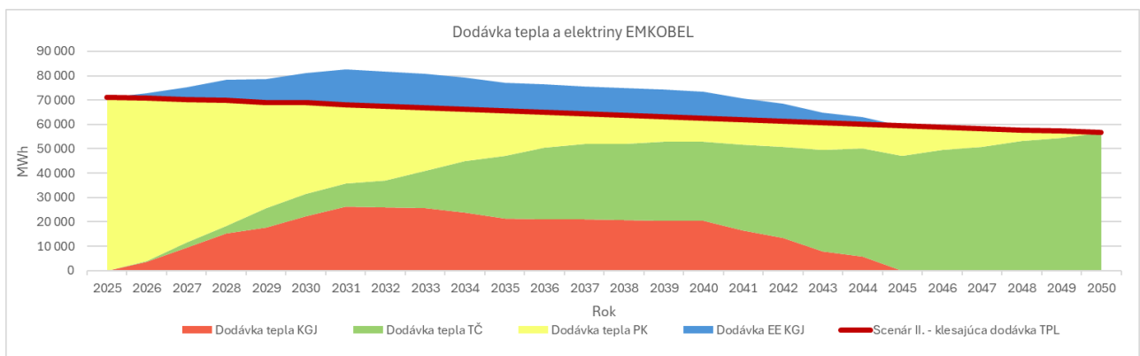
Obr. 61: Energetické vstupy EMKOBEL – scenár 2 klesajúci o 1%
