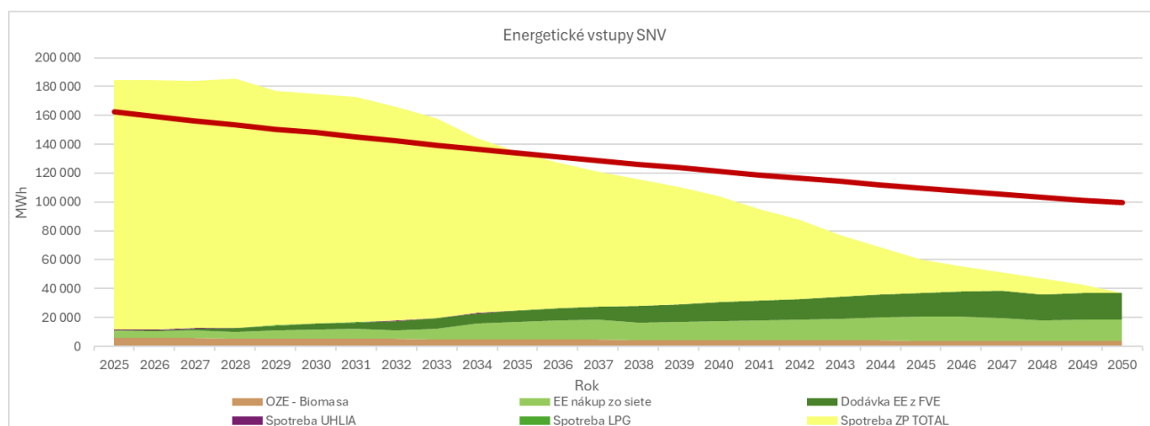
Obr. 79: Energetické vstupy - celá SNV - scenár 3 klesajúci o 2%
