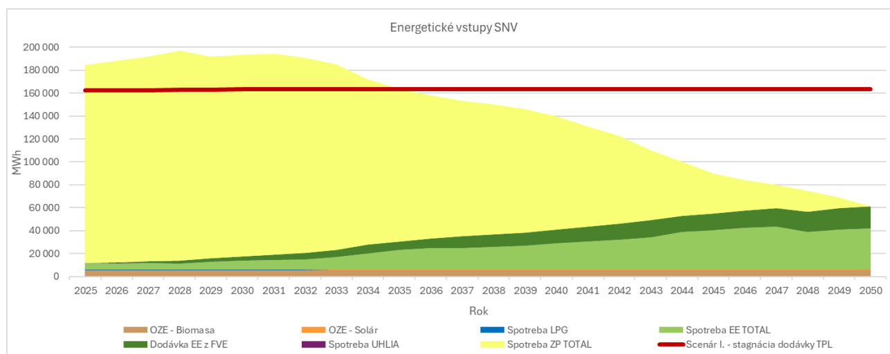
Obr. 55: Energetické vstupy - celá SNV - scenár 1 stagnačný
