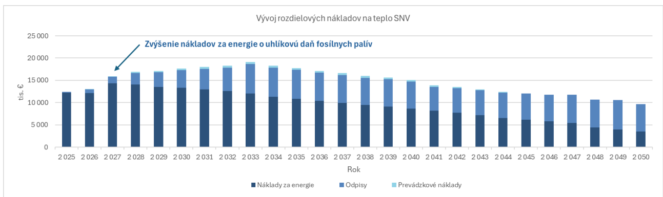
Obr. 68: Vývoj rozdielových nákladov na teplo - celá SNV - scenár 2 klesajúci o 1%
